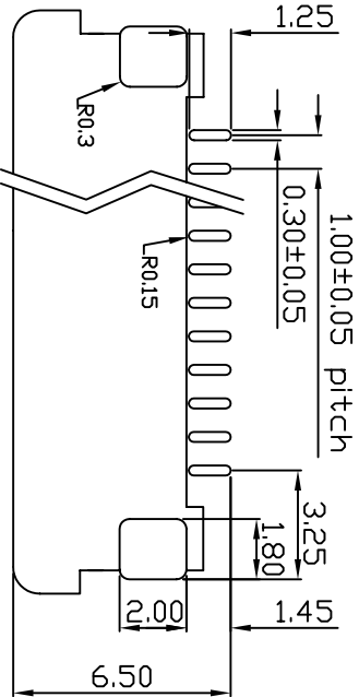
P.C.B Layout
