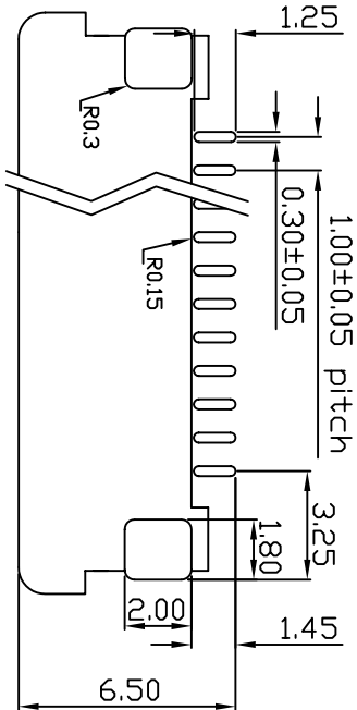
P.C.B Layout
